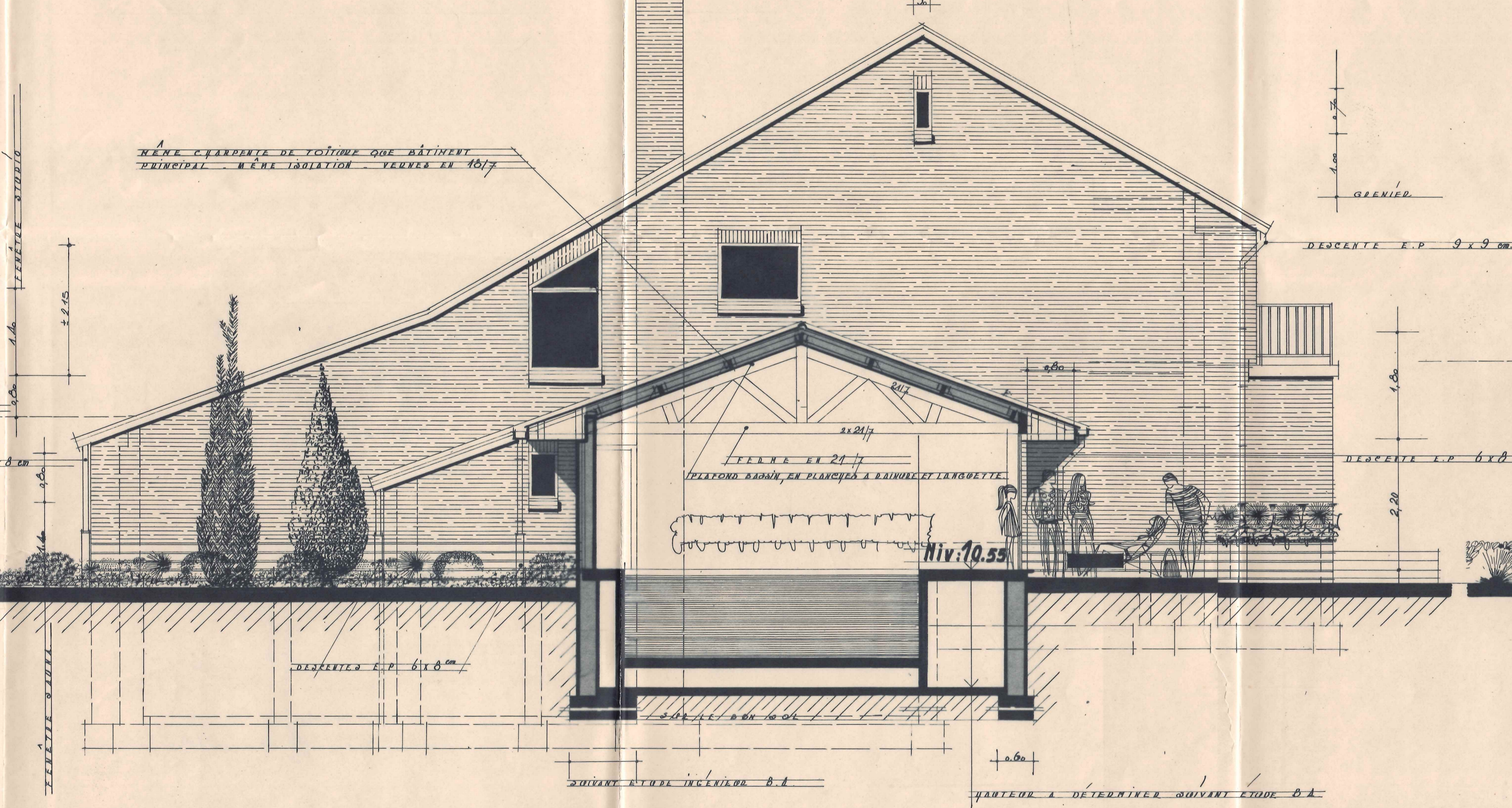
COUPE DANS BASSIN
